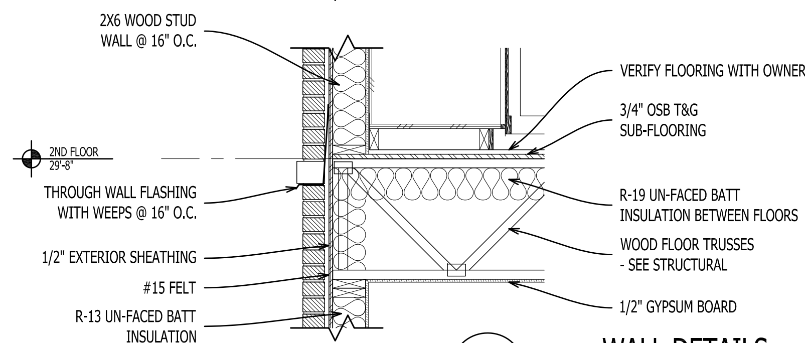
2 A-501 WALL DETAILS Scale: 3/4" = 1'-0"
