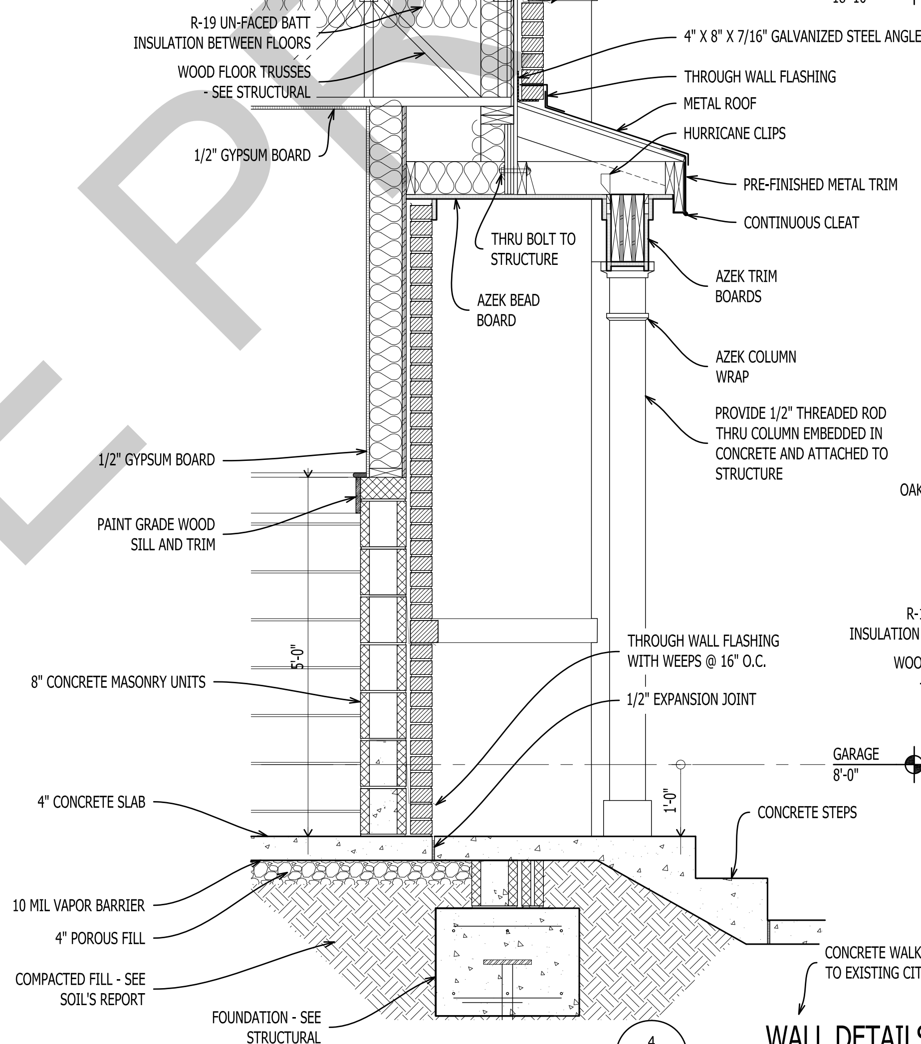
5 A-501 WALL DETAILS Scale: 3/4" = 1'-0"
