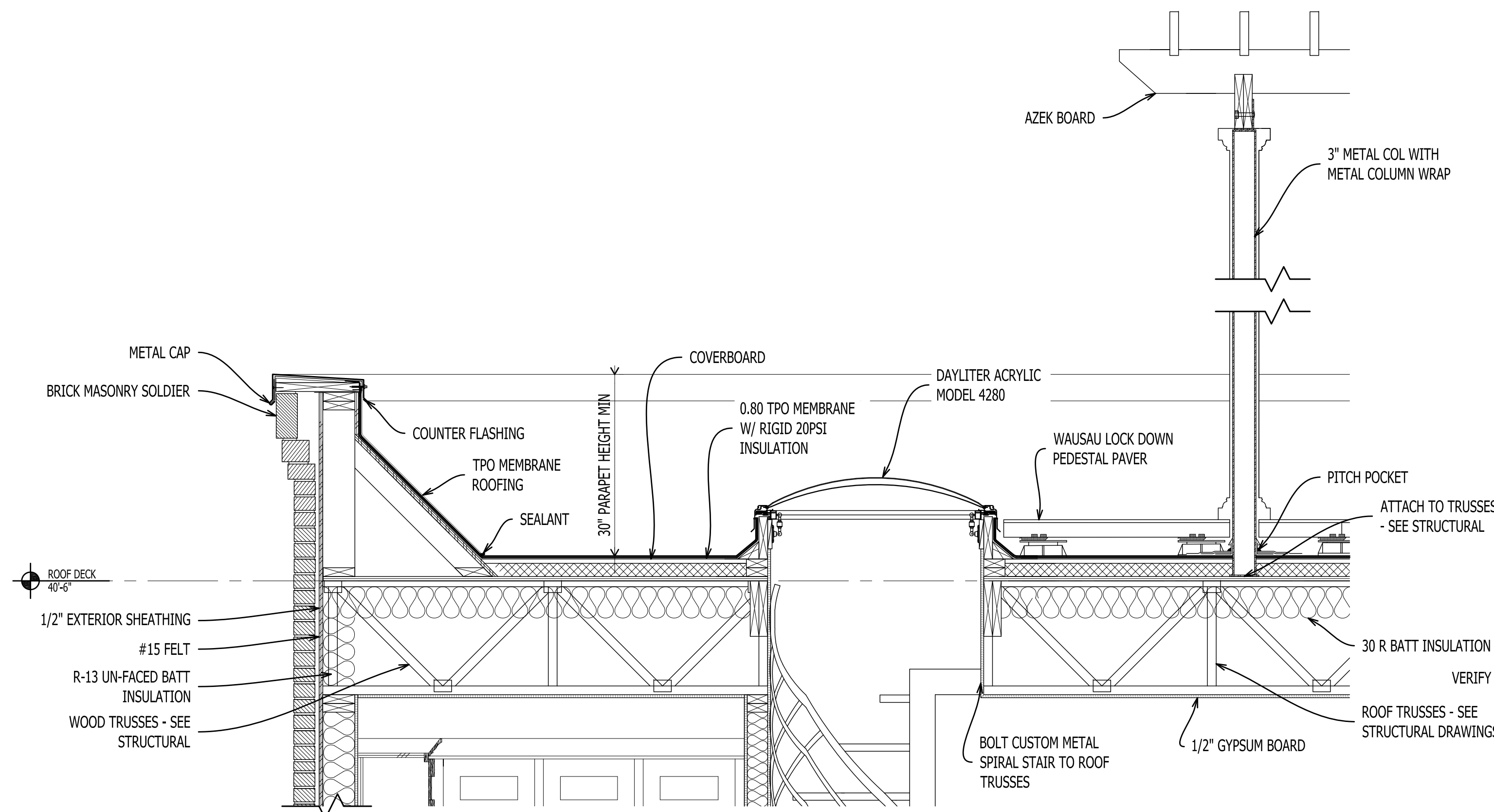
3 A-501 WALL DETAILS Scale: 3/4" = 1'-0"
