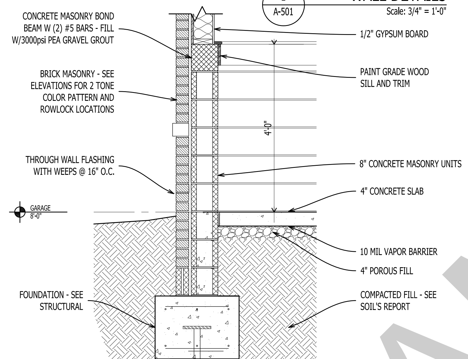
1 A-501 WALL DETAILS Scale: 3/4" = 1'-0"
