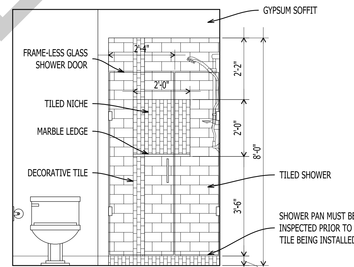
7 A-401 SHOWER ELEVATION Scale: 1/2" = 1'-0"
