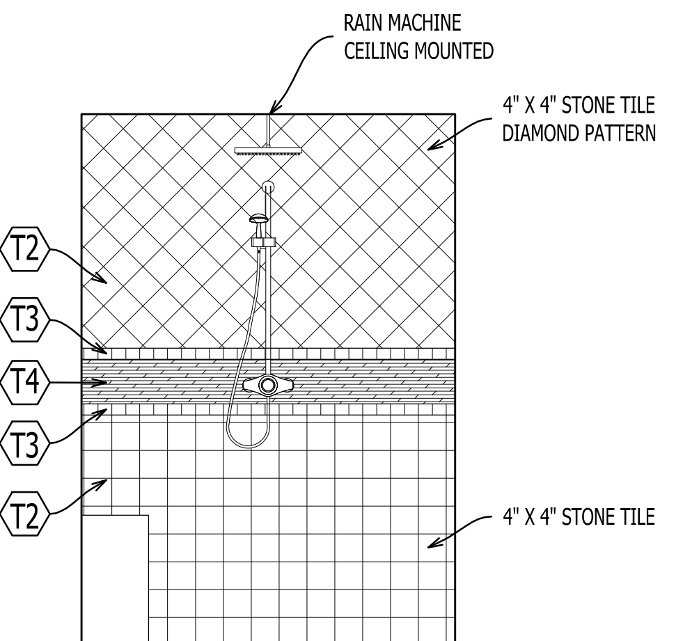
4 A-201 SHOWER ELEVATION Scale: 1/2" = 1'-0"
