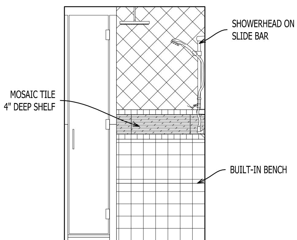
3 A-201 SHOWER ELEVATION Scale: 1/2" = 1'-0"
