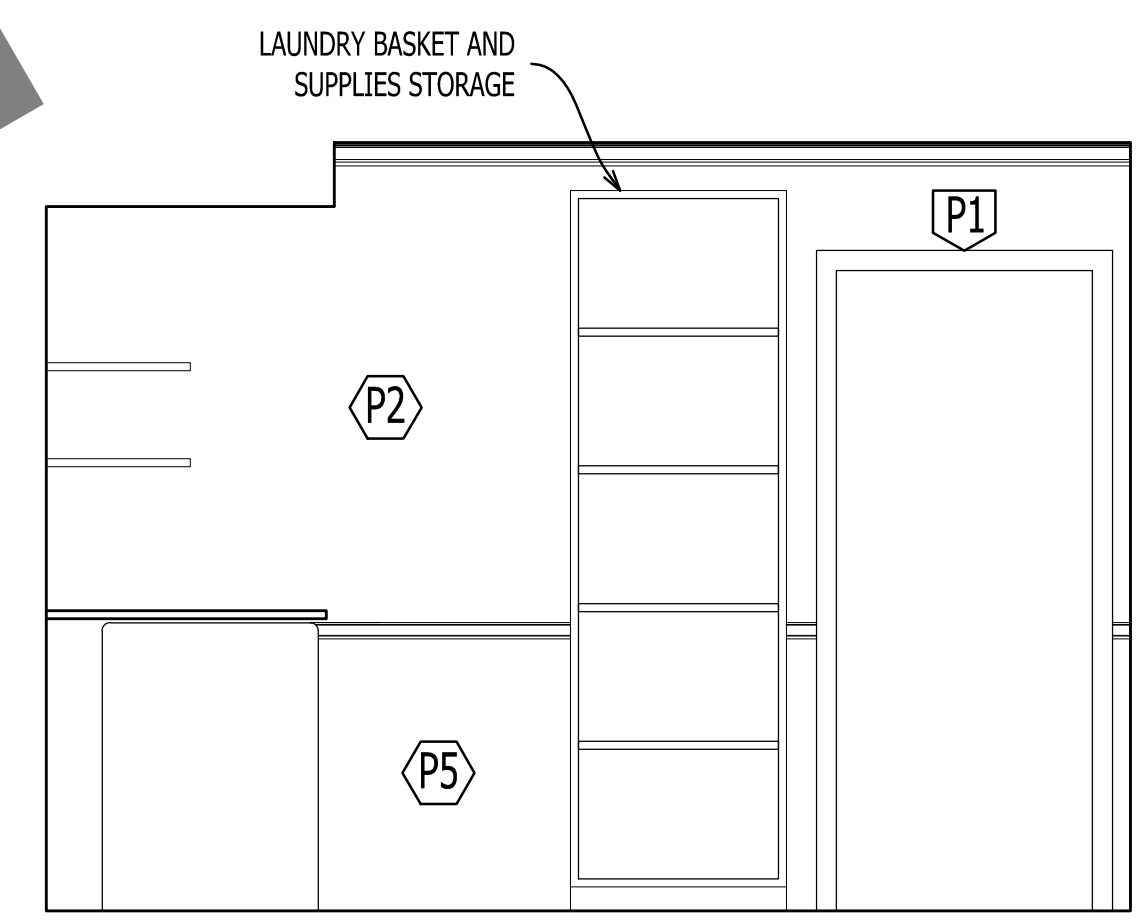
1 A-201 LAUNDRY ELEVATION Scale: 1/2" = 1'-0"
