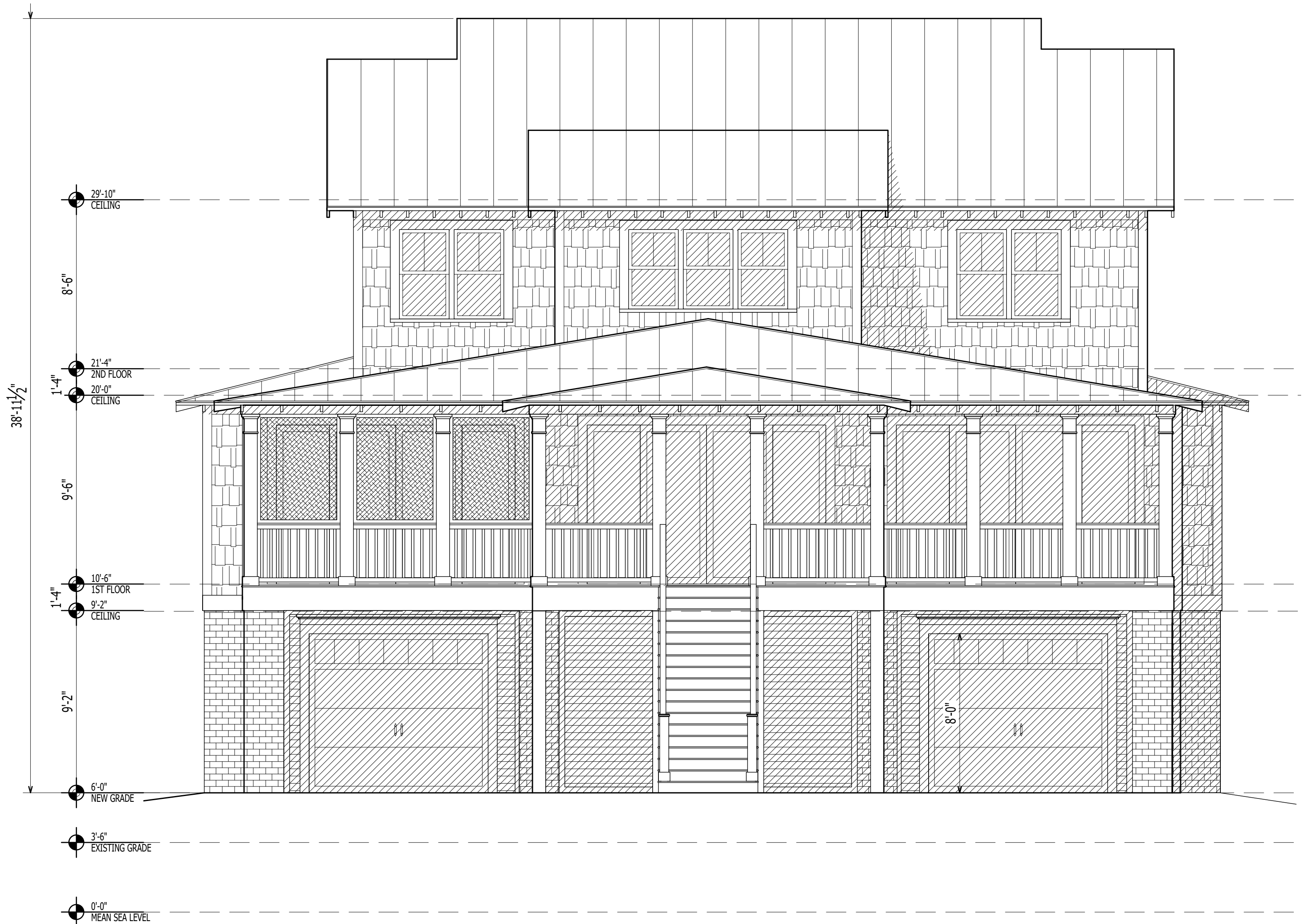
2 A-201 ELEVATION Scale: 1/4" = 1'-0"
